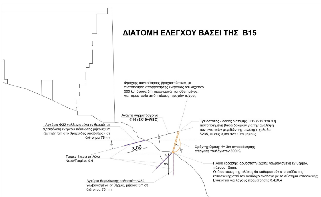
Εικόνα 3: Περιοχή VI - Διατομή
