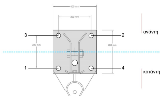
Εικόνα 6: Περιοχή IV - Λεπτομέρεια θεμελίωσης
