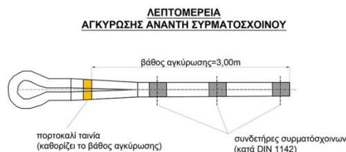
Εικόνα 7: Λεπτομέρεια αγκύρωσης ανάντη συρματόσχοινου
