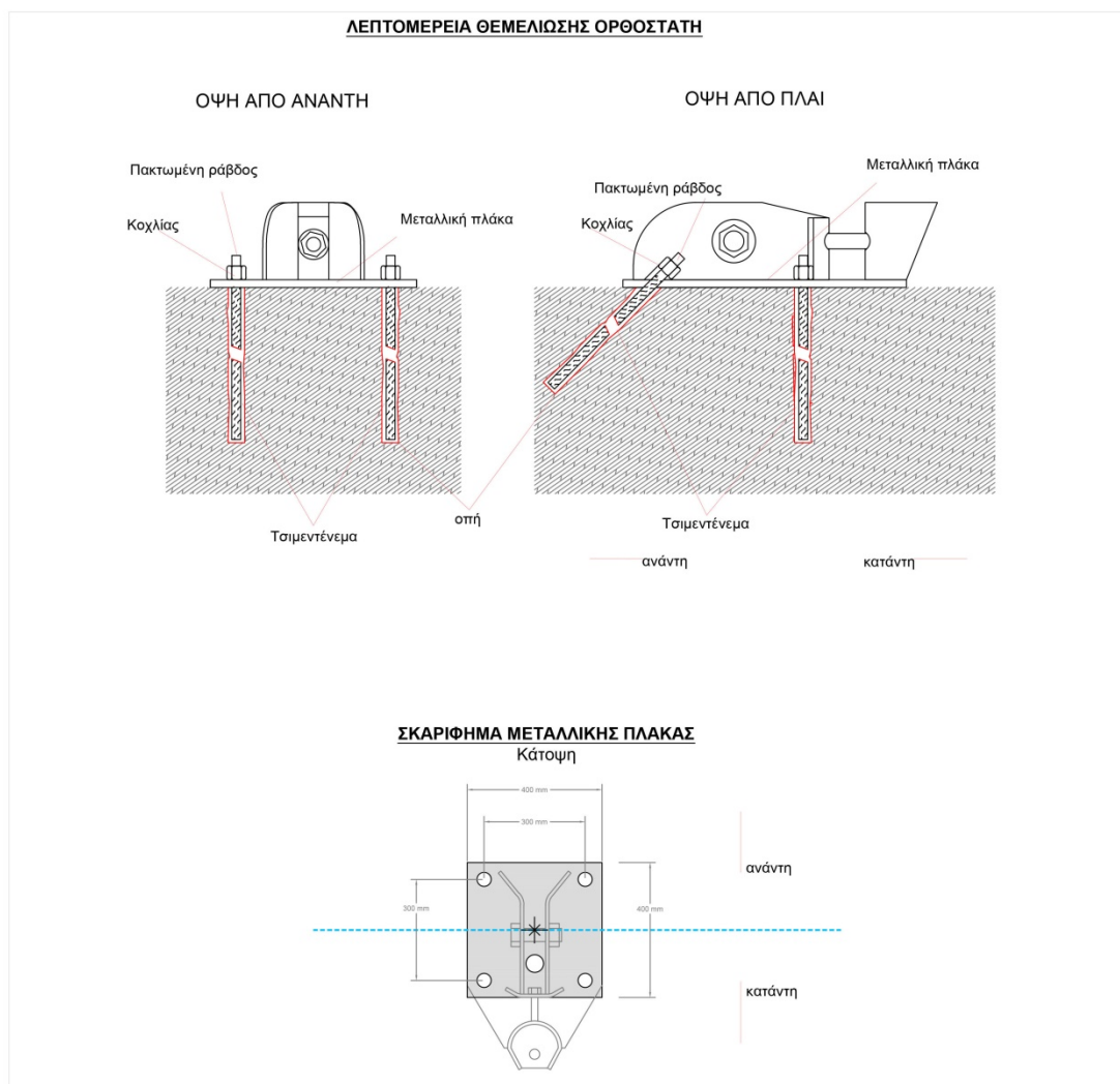
Εικόνα 5: Περιοχή VI - Λεπτομέρεια θεμελίωσης
