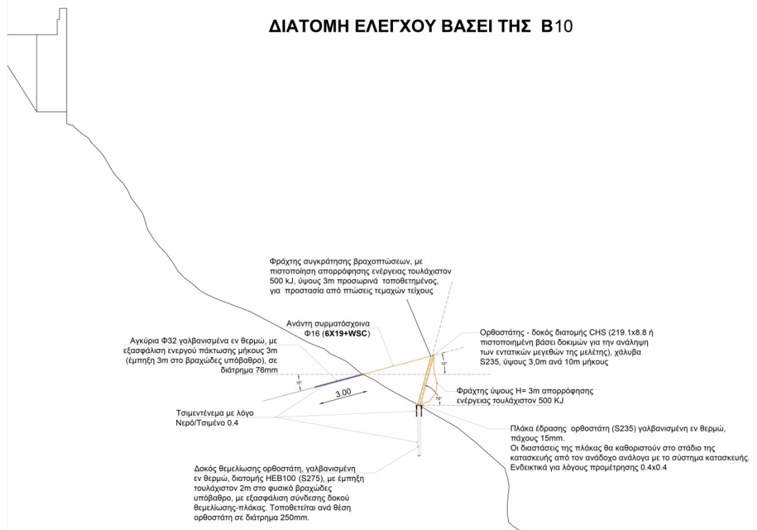
Εικόνα 2: Περιοχή IV - Διατομή
